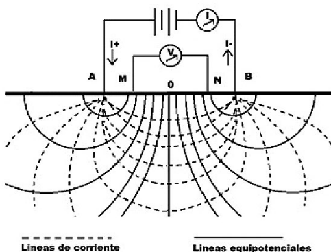
Fig. 1 Esquema básico de dispositivo para determinar la resistividad eléctrica del subsuelo.
